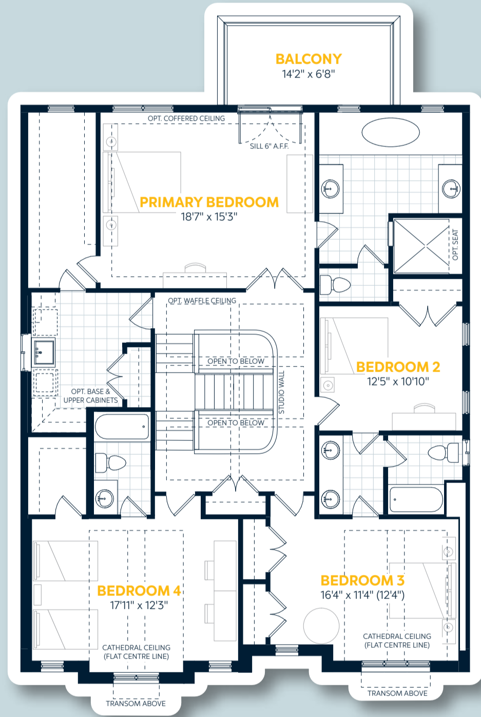
Elevation B
