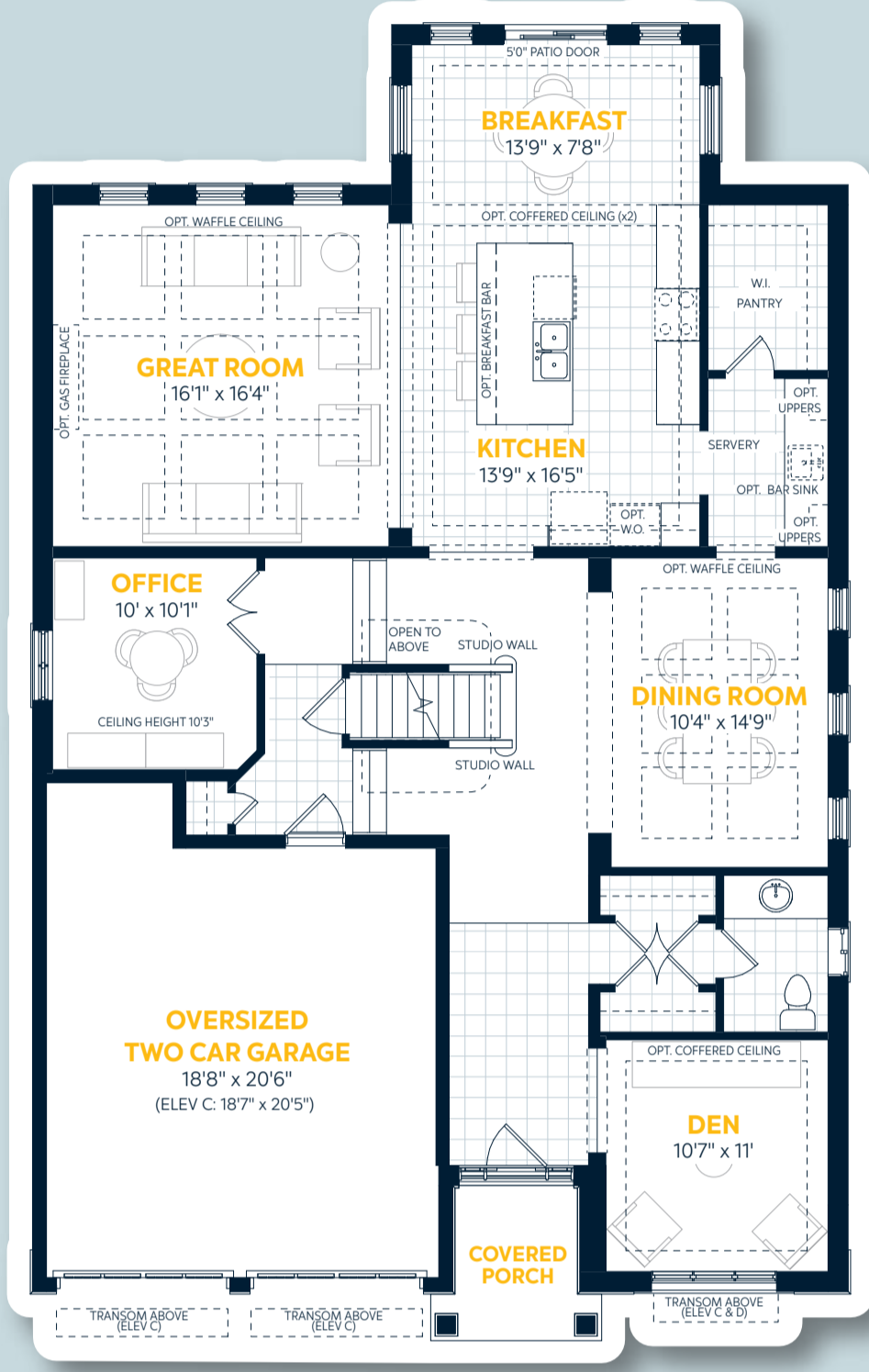
Elevation B
